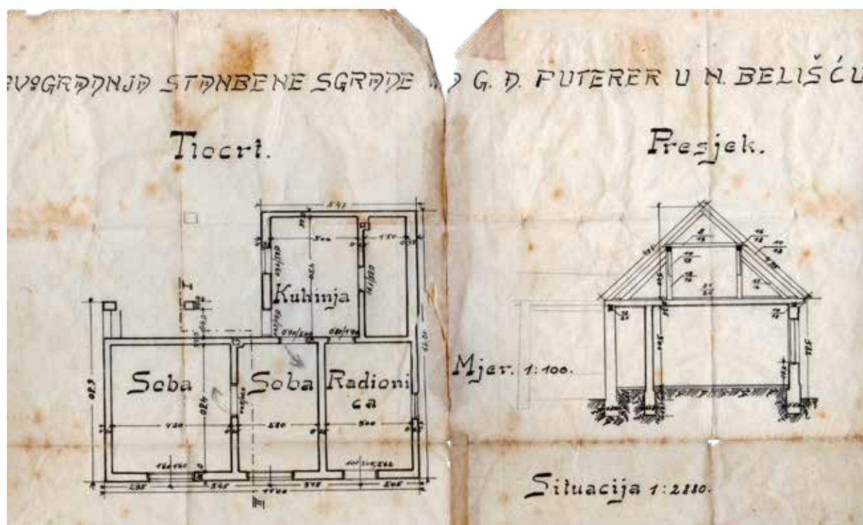
Slika 20 a. Tlocrt i presjek kuće za G. Đ. Putterera (vlasnik dokumenta Dubravko Maričić – privatni arhiv)
